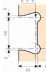
Für 3 mm Luft For 3 mm gap
