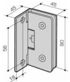
Für 5 mm Luft For 5 mm gap
