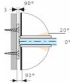
Glas/Wand 3 oder 5 mm Glass/Wall 3 or 5 mm
