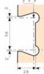
Für 5 mm Luft For 5 mm gap
