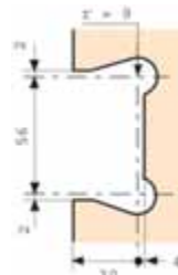
Für 3 mm Luft For 3 mm gap
