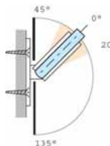
Glas/Wand 3 mm Luft Glass/Wall 3 mm gap
