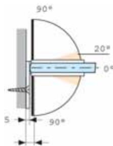
Glas/Wand 3 oder 5 mm Glass/Wall 3 or 5 mm
