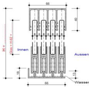
WS 8 4 bahnig / 4 teilig
