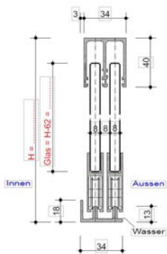
WS 8 2 bahnig / 2 teilig
