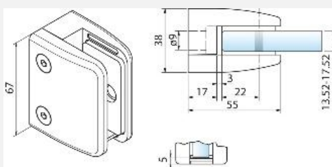
Klemmhalter 4893ZN22 55x67mm für 16mm Edelstahlfinish
