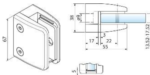
Klemmhalter 4891ZN22 55x67mm für 12mm Edelstahlfinish
